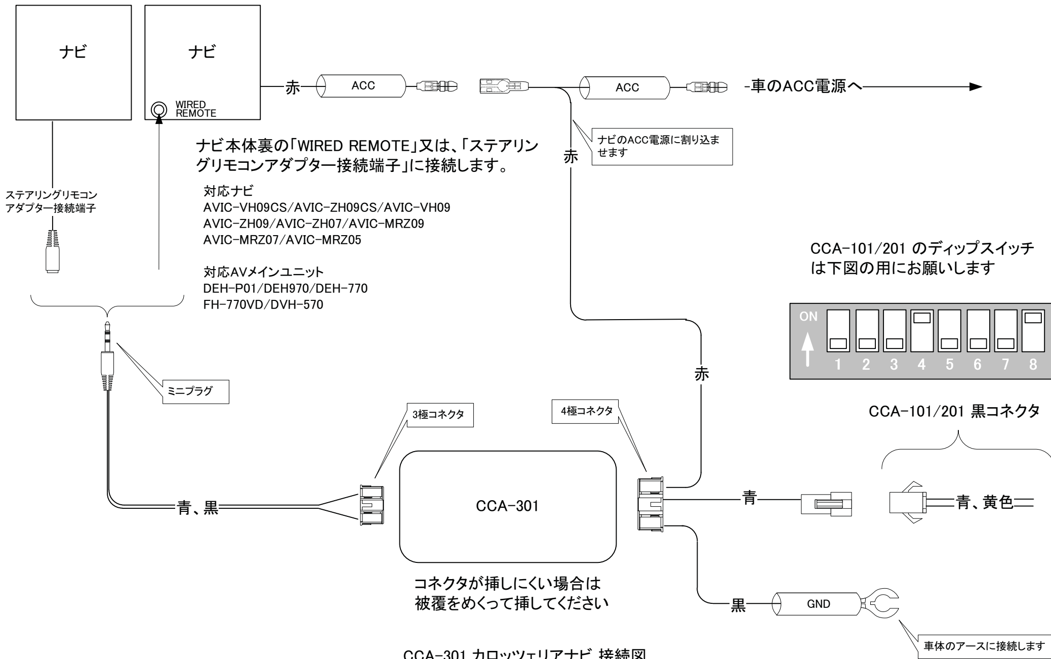
CCA-301 カロッツェリアナビ 接続図
