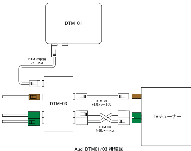
Audi DTM01/03 接続図
