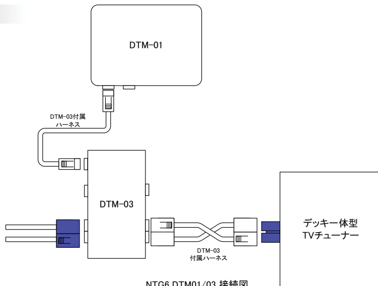
NTG6 DTM01/03 接続図
