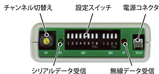
スイッチ面
