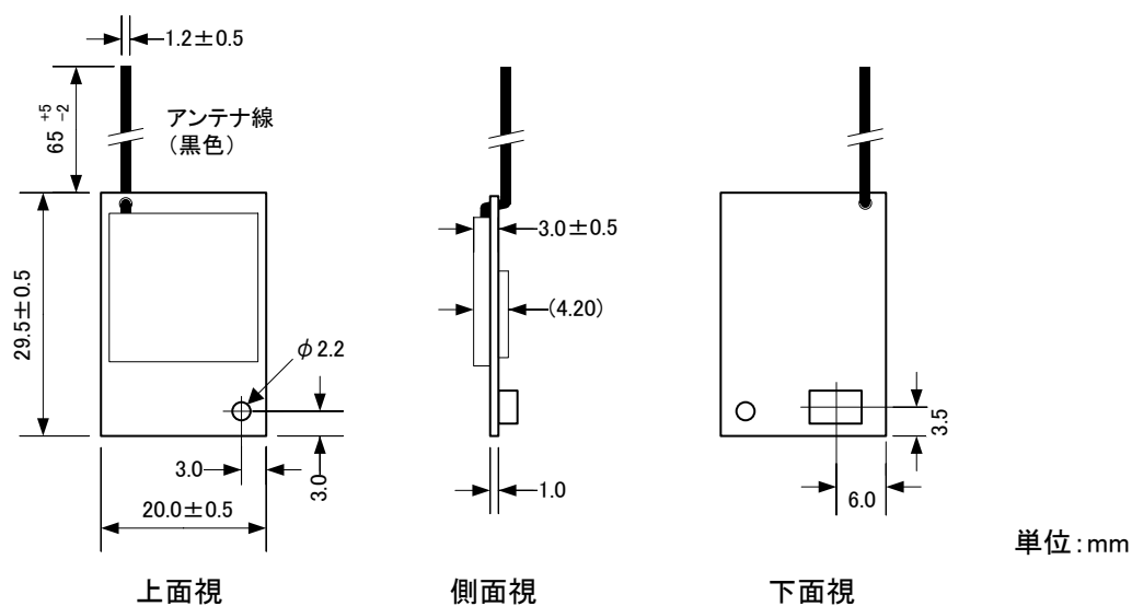
図8 外形寸法図
